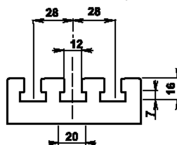
velikost "T" drážky
