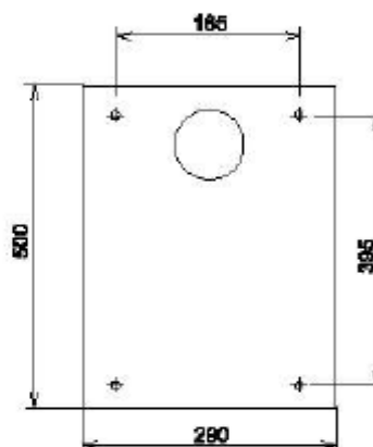
Rozteče děr v základně
