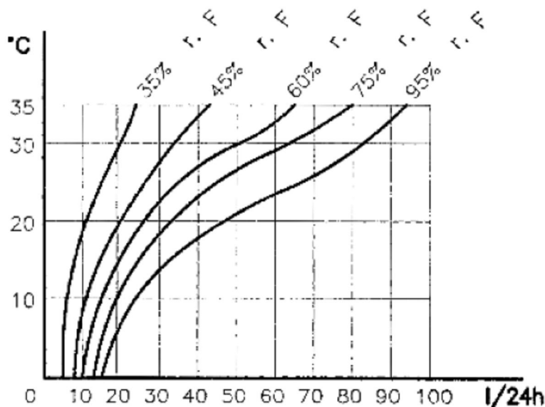
Diagram výkonu T 97/95
