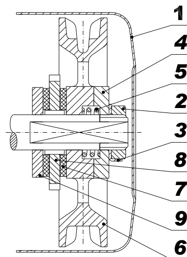
Obr. 11.3 - Seřízení brzdy
